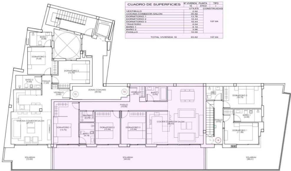
PLANTA ATICO 4
